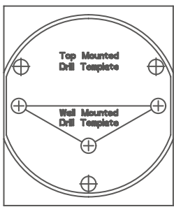
Πρότυπο διάτρησης (×1)
