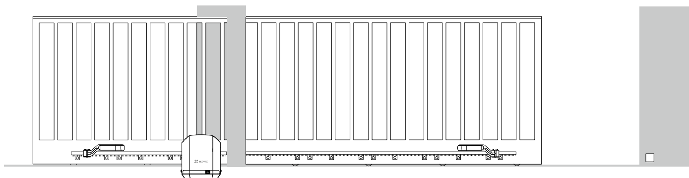
Αριστερή Εγκατάσταση
