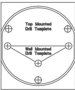
Πρότυπο διάτρησης (×1)
