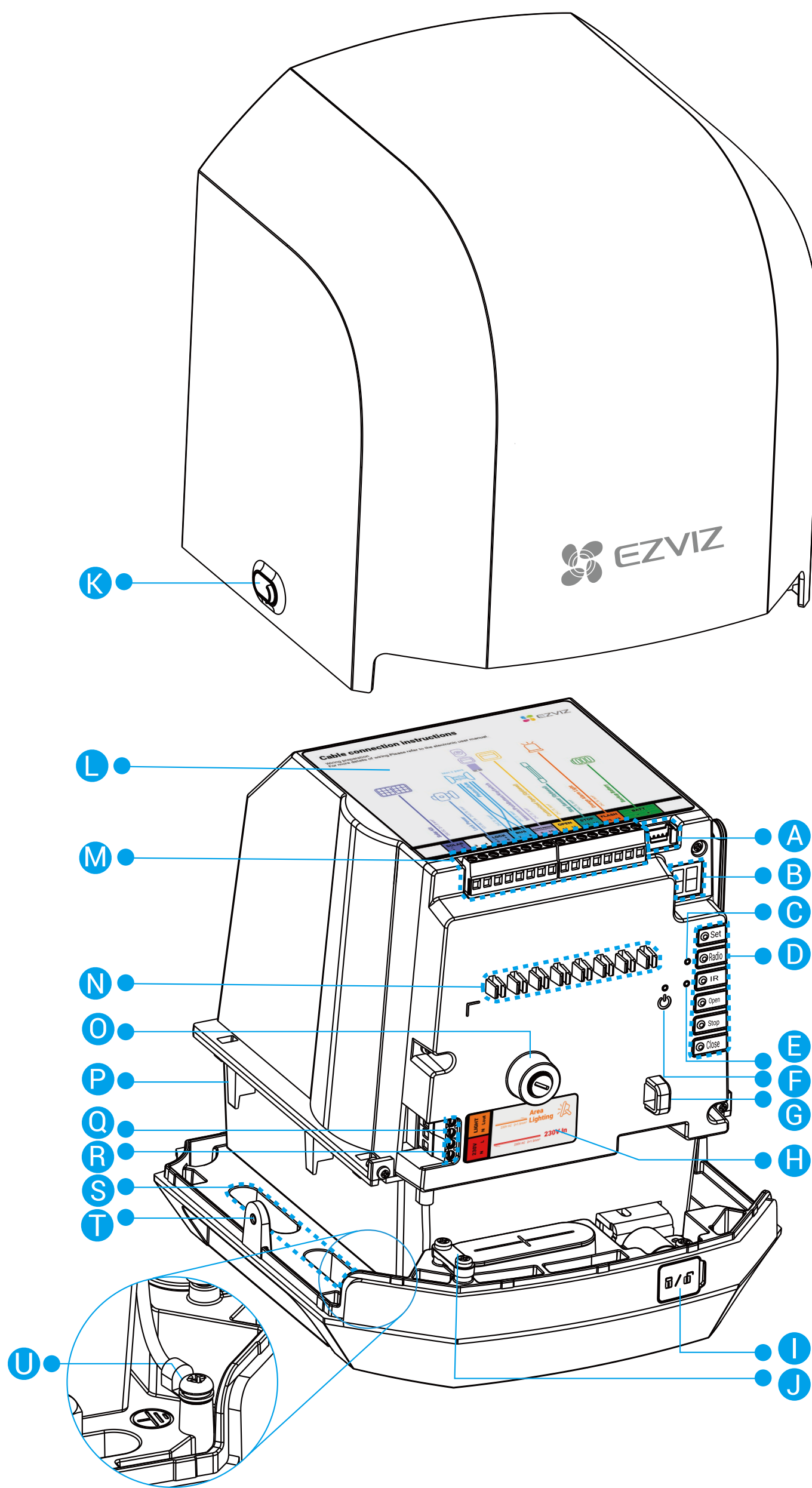
Προβολή μπροστά
